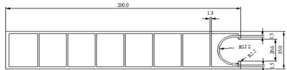
8202 PERFIL TAPON ADAPTADOR POSTE
