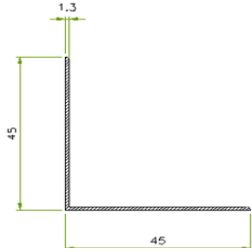
8013 CANTONERA 45X45 (RECOGE GOTAS)
