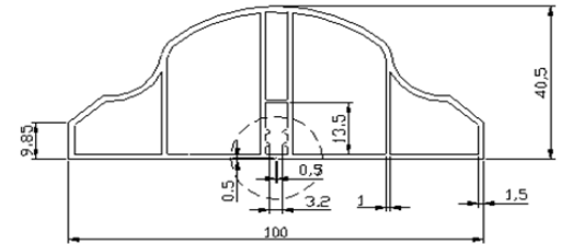
8034 PERFIL VALLA CONVEXO
