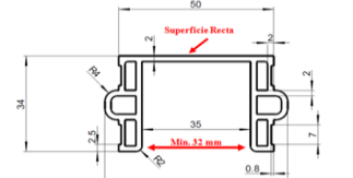
8202 PERFIL TAPON ADAPTADOR POSTE
