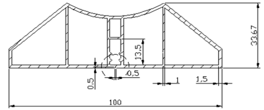
8034 PERFIL VALLA CONVEXO
