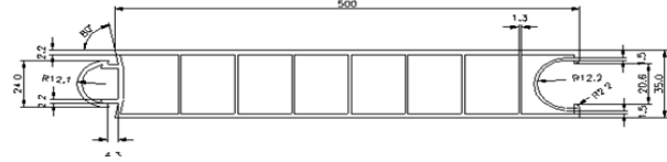
8092 EXPANEL DE 500 LM
